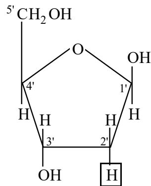
Deoxyribose
